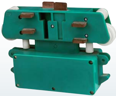
弧形 10-10/50 MG-H010
